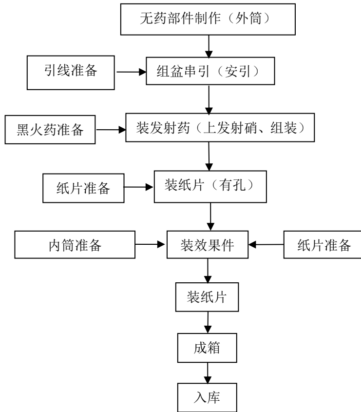
图 2.4-3 组合烟花产品生产工艺流程图
