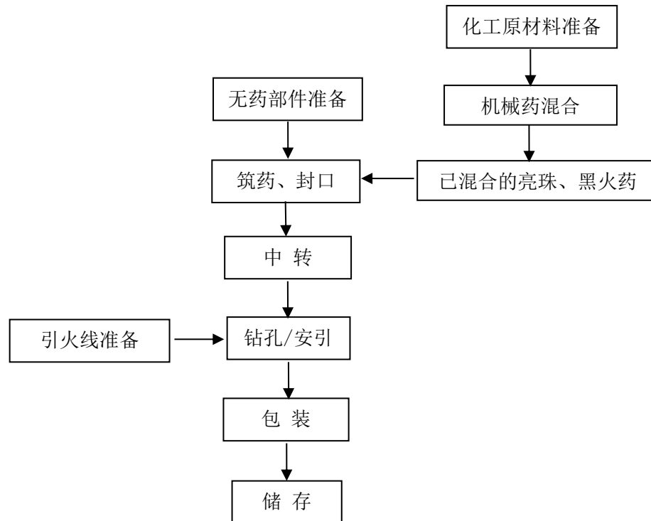
图 2.4-5 喷花类产品生产工艺流程图
